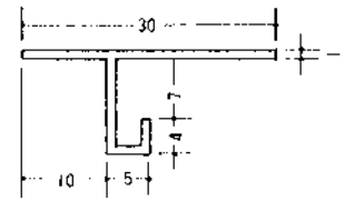
AM-6 (B2アルマイト)3m
