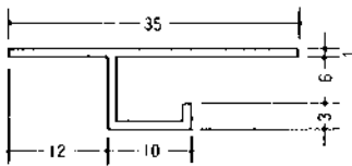
AZ-7K (B2アルマイト)3m
