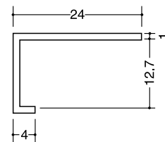
KTC-13 (B2アルマイト) 3m
