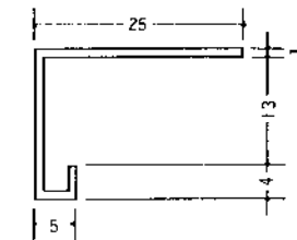
KTC-7 (B2アルマイト) 3m
