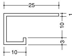
AC-10K (B2アルマイト) 3m
