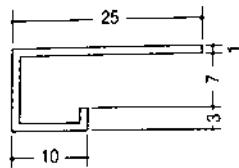
AC-7K (B2アルマイト) 3m
