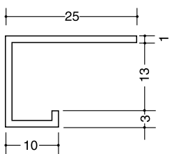
AC-13K (B2アルマイト) 3m
