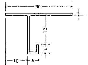
AM-12 (B2アルマイト)3m
