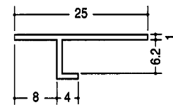
KMA-6 (B2アルマイト)3m
