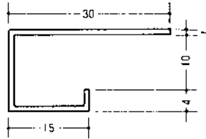
A型13 (B2アルマイト) 3m
