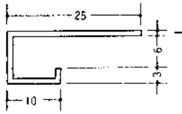
AC-7K (B2アルマイト) 3m
