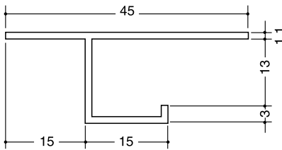
アルミB型16 (B2アルマイト)3m
