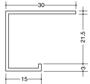
A型20 (B2アルマイト) 3m
