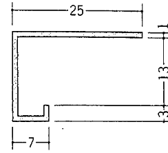
KCD-12 (B2アルマイト)3m
