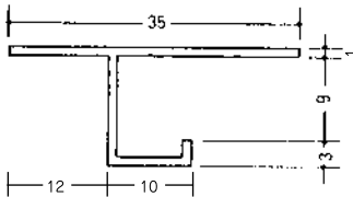
AZ-9K (B2アルマイト)3m
