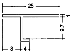
KMA-9 (B2アルマイト)3m
