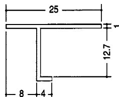
KMA-12 (B2アルマイト)3m
