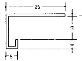
CC-9 (B2アルマイト) 3m
