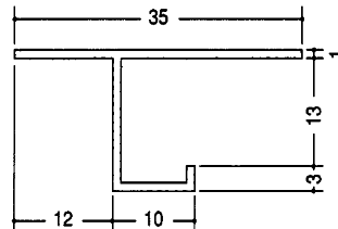
KMA-12 (B2アルマイト)3m
