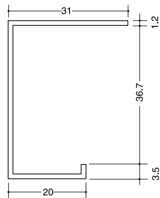
A型36 (B2アルマイト) 3m
