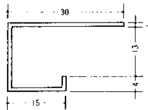
A型13 (B2アルマイト) 3m
