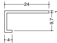
KTC-10 (B2アルマイト) 3m
