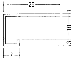
KCD-9 (B2アルマイト)3m
