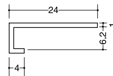
KTC-7 (B2アルマイト) 3m
