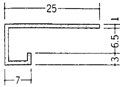
KCD-6 (B2アルマイト)3m
