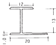
13HS (2.73m)
