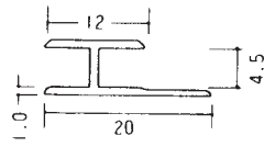
4.5HS (2.73m)
