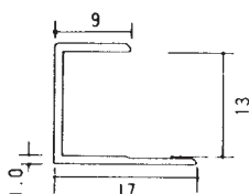
13CS (2.73m)
