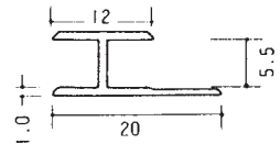
5.5HS (2.73m)
